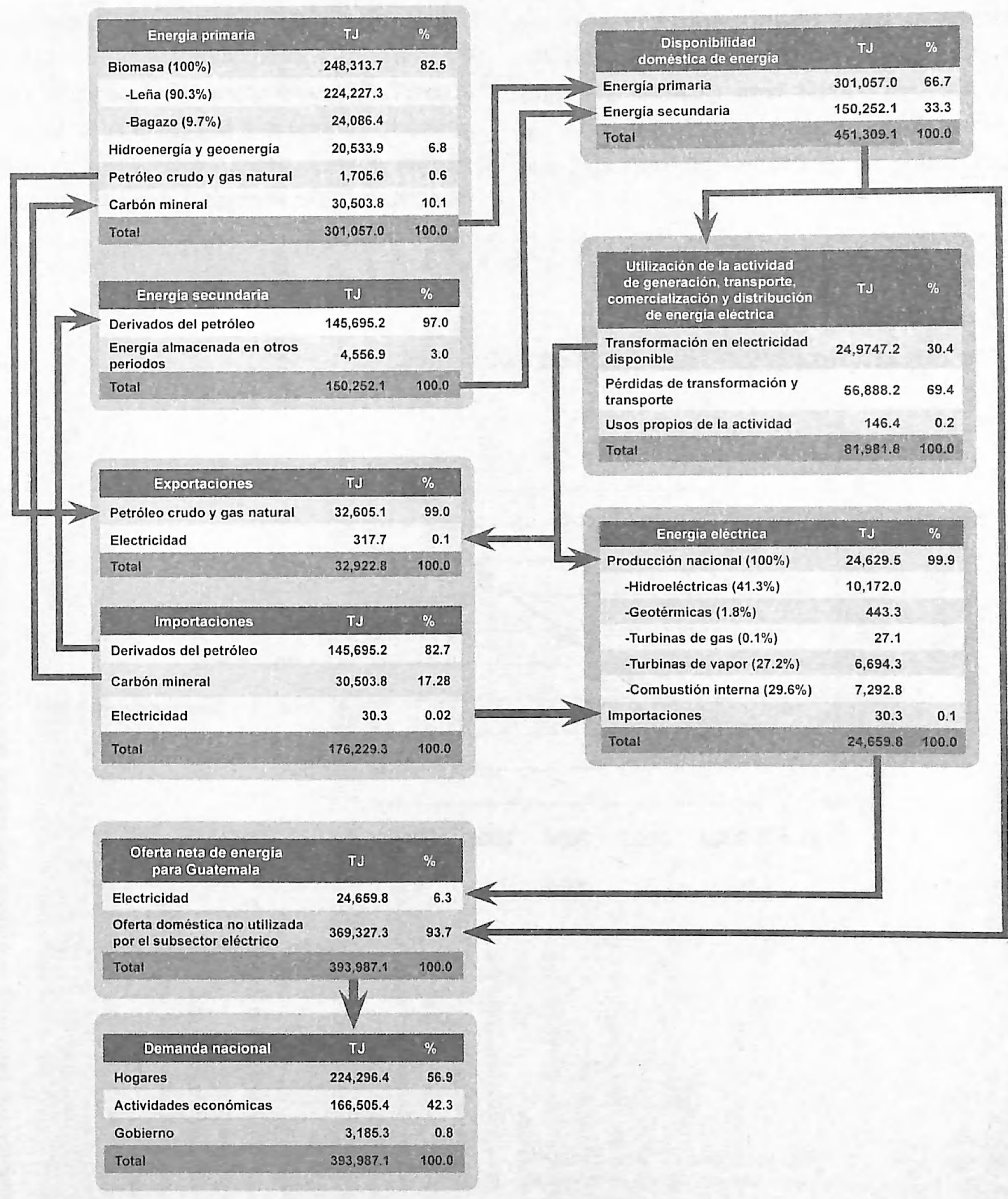
Esquema de los flujos energéticos en Guatemala para el año 2006
